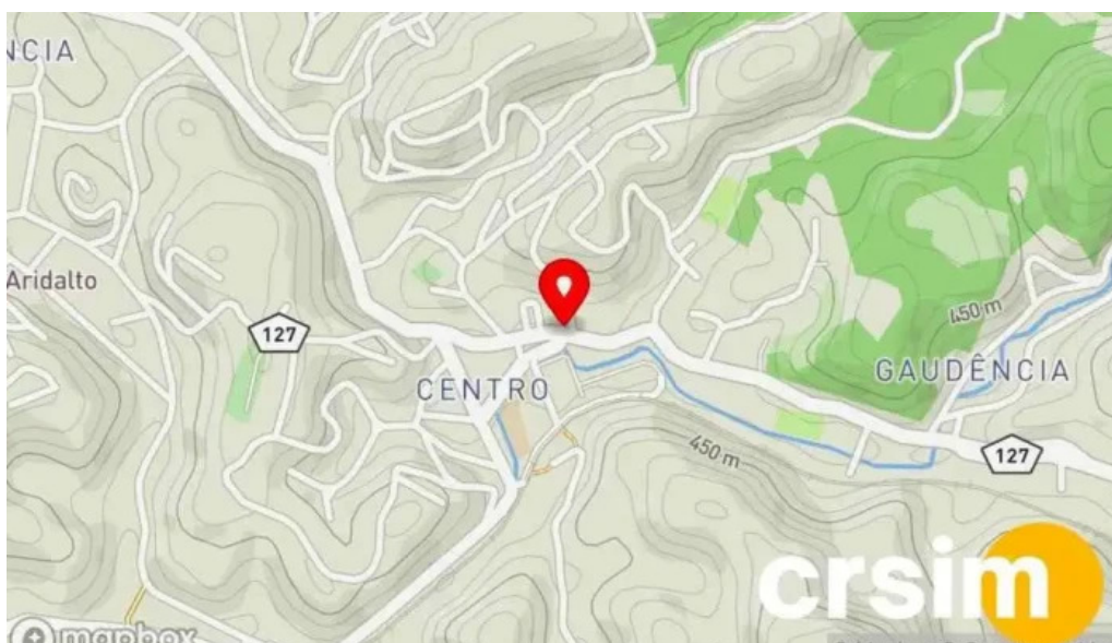
Mendes mapa
